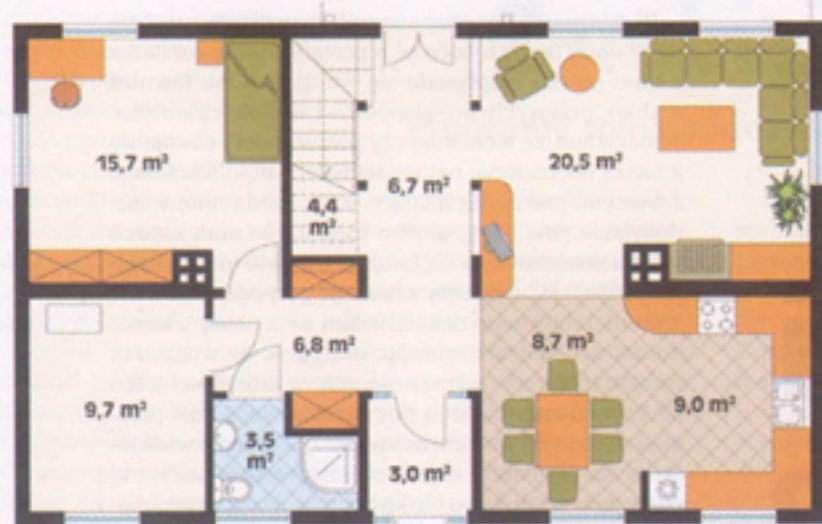
Rzut parteru
